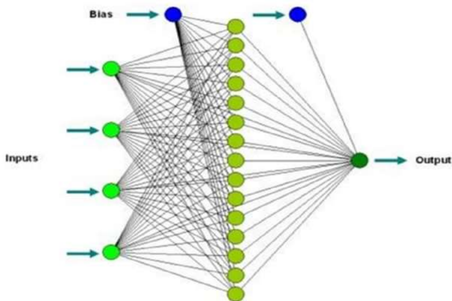
شکل ۱- شبکه عصبی چندلایه پیش‌رو
